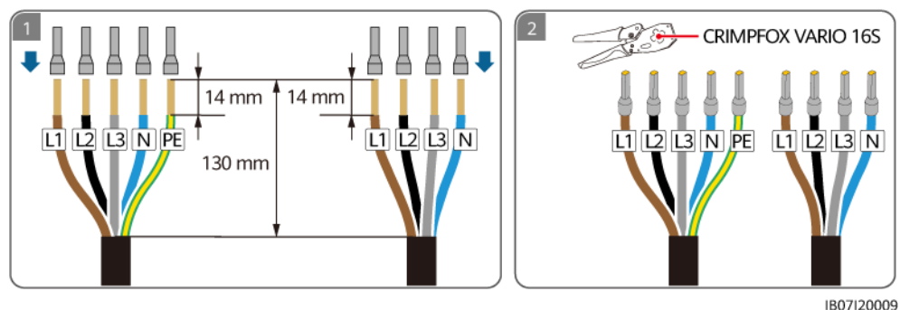
Abbildung 5-17 Crimpen der AC-Kabelendklemmen
