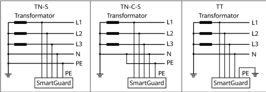
Abbildung 2-7 Erdungssysteme
