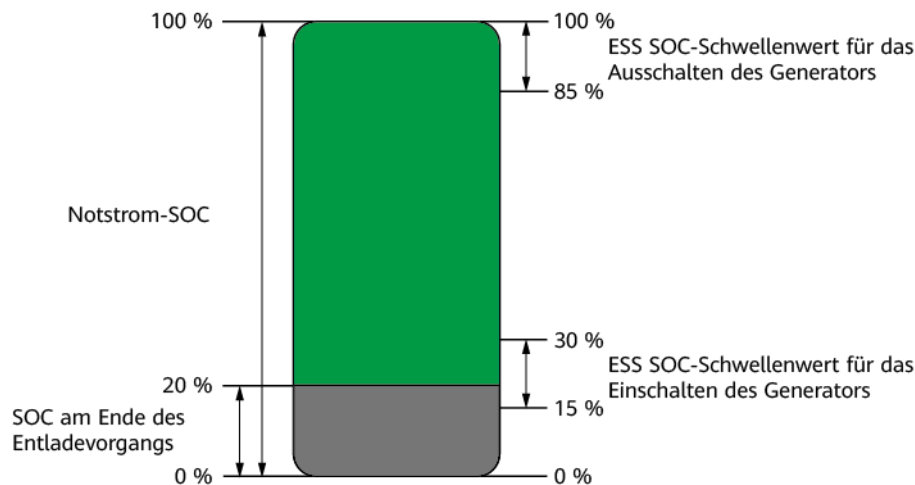
Abbildung 6-15 Batterie-SOC
